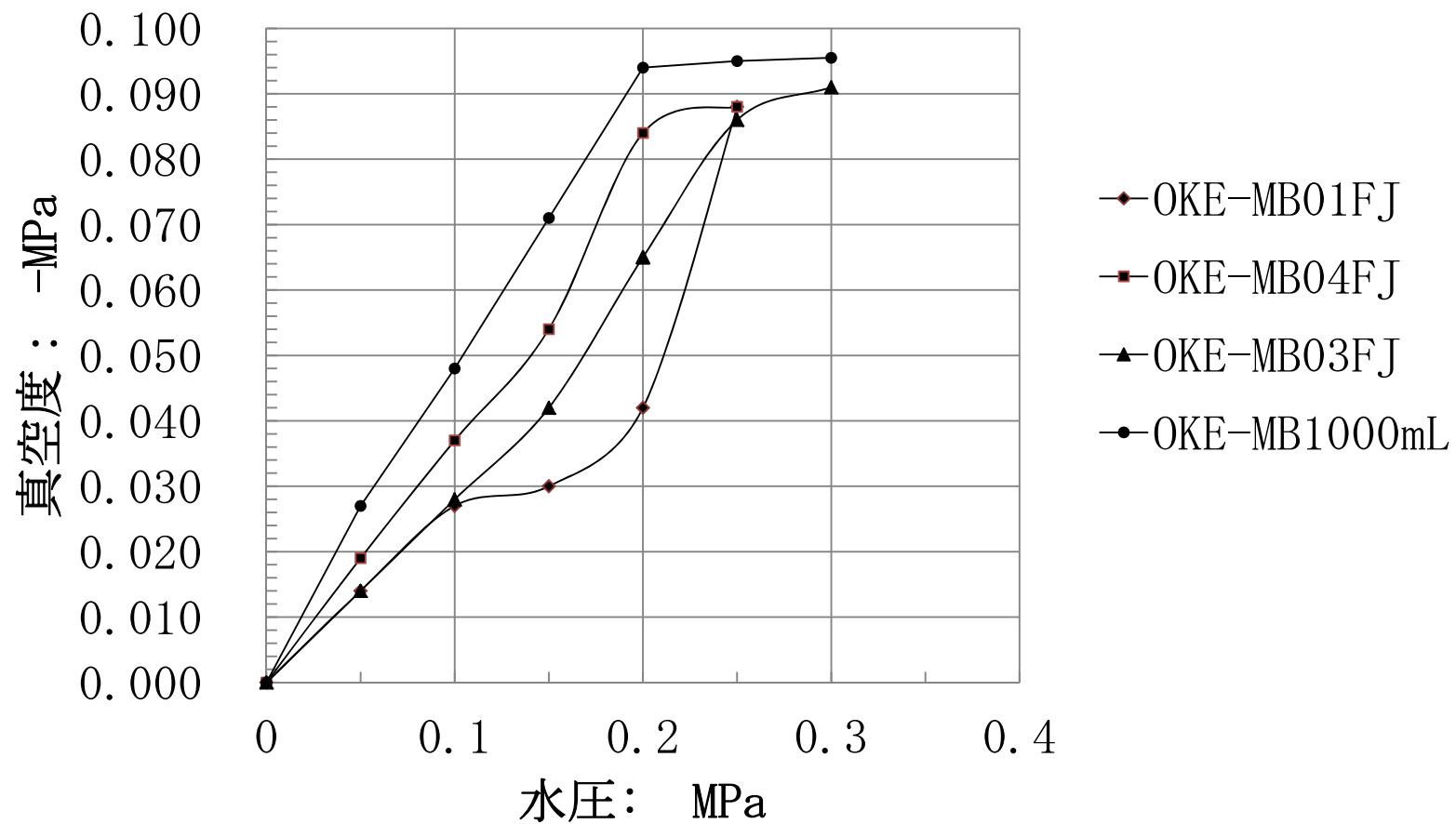
ノズル4種類の真空度比較
